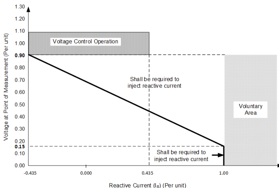
รูปที่ O-16 การควบคุมการจ่ายหรือรับ Reactive Current ของผู้เชื่อมต่อที่ใช้อุปกรณ์ Inverter
