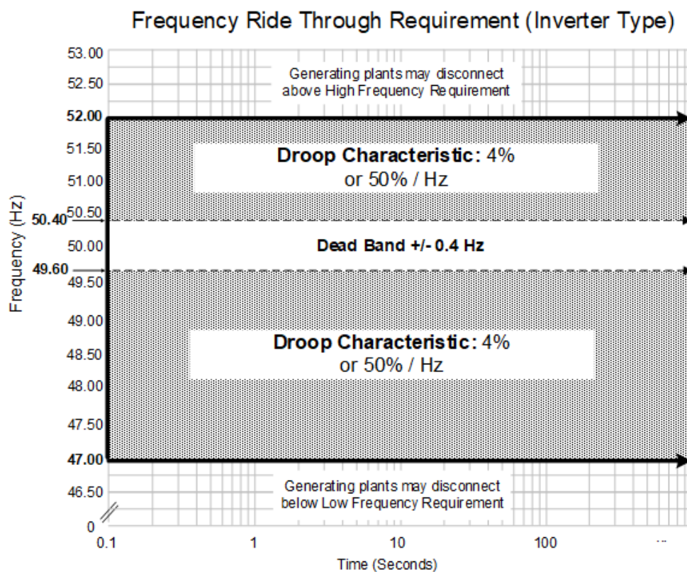
รูปที่ O-19 เกณฑ์ Frequency Ride Through ของโรงไฟฟ้าที่ใช้อุปกรณ์ Inverter
