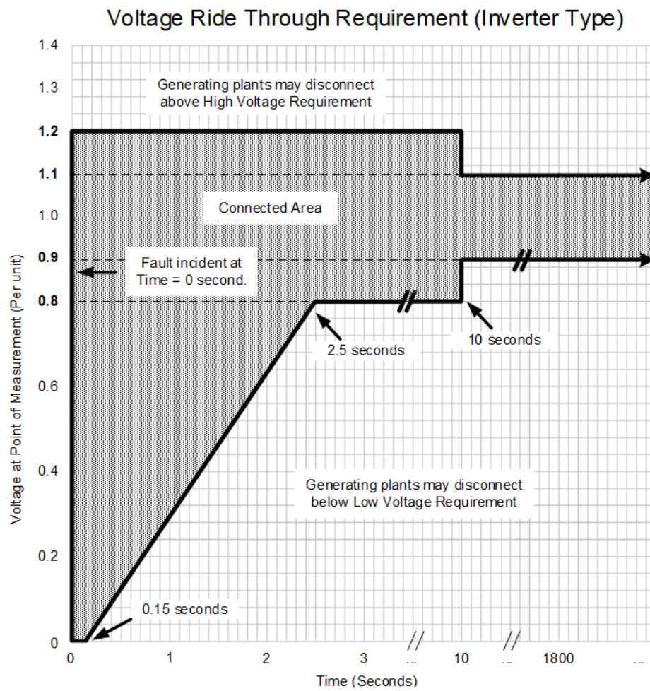
รูปที่ O-9 เกณฑ์ Voltage Ride Through ของ BESS
