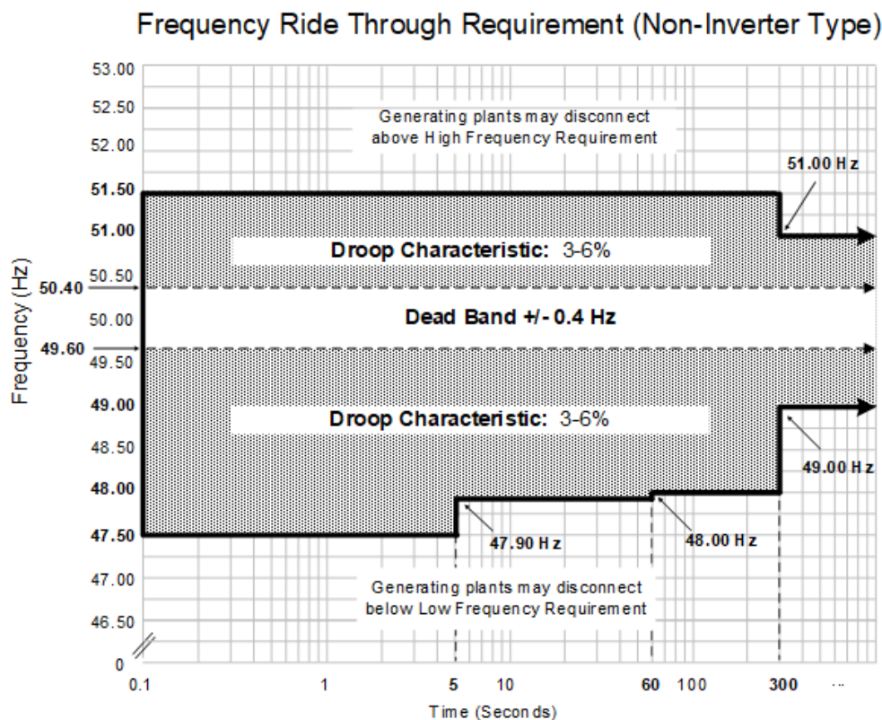
รูปที่ O-12 เกณฑ์ Frequency Ride Through ของโรงไฟฟ้าที่ไม่ใช้อุปกรณ์ Inverter
