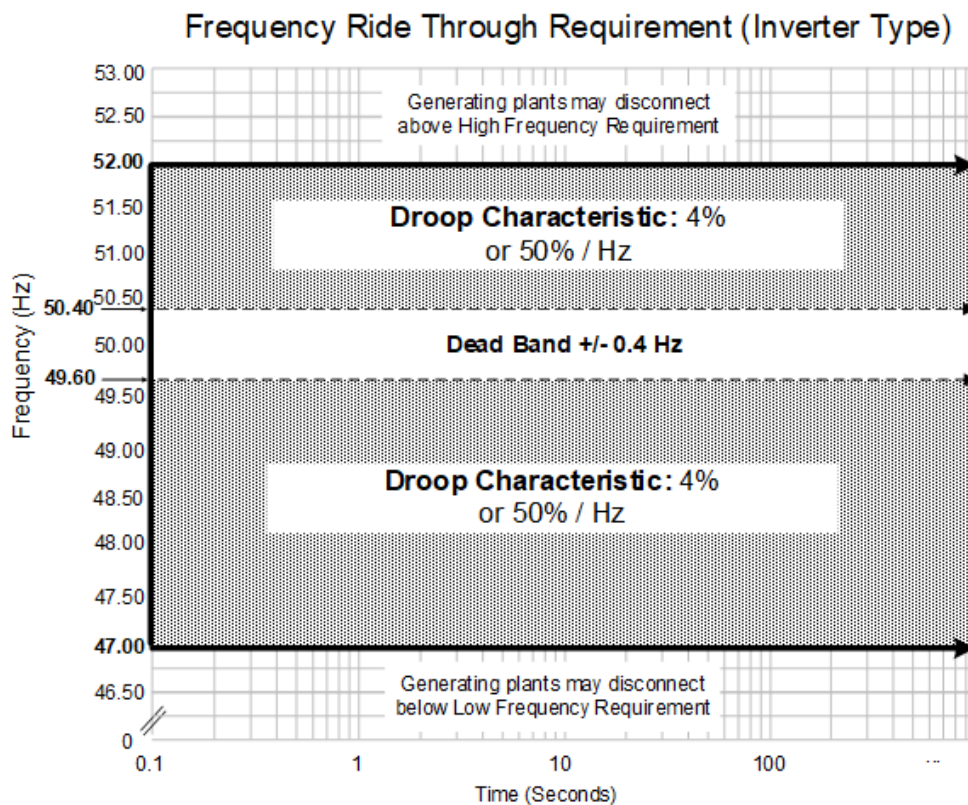
รูปที่ O-14 เกณฑ์ Frequency Ride Through ของโรงไฟฟ้าที่ใช้อุปกรณ์ Inverter
