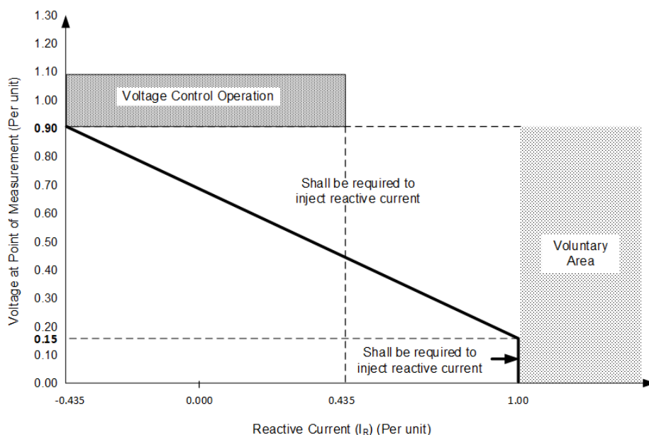
รูปที่ O-5 การควบคุมการจ่ายหรือรับ Reactive Current ของผู้เชื่อมต่อที่ใช้อุปกรณ์ Inverter
