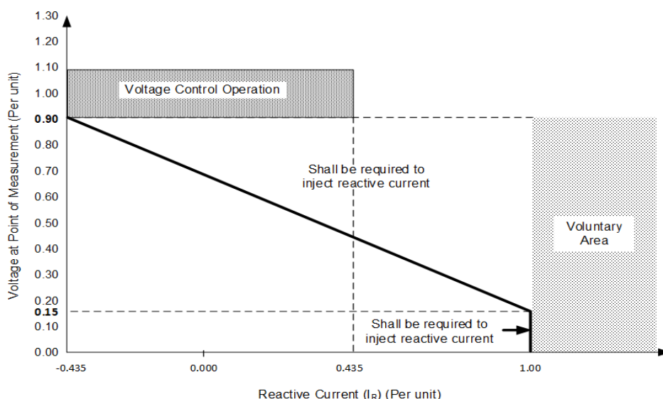
รูปที่ O-21 การควบคุมการจ่ายหรือรับ Reactive Current ของผู้เชื่อมต่อที่ใช้อุปกรณ์ Inverter
