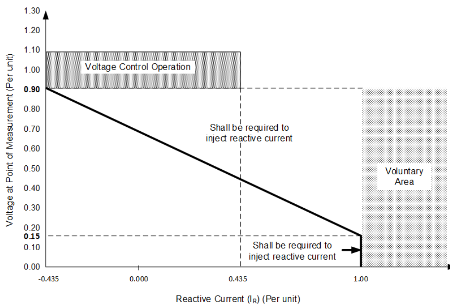
รูปที่ O-10 การควบคุมการจ่ายหรือรับ Reactive Current ของผู้เชื่อมต่อที่ใช้อุปกรณ์ Inverter
