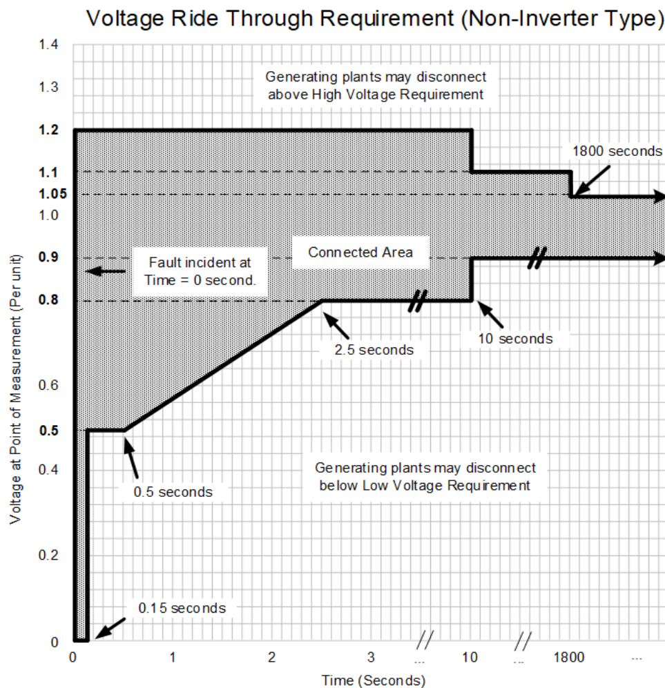
รูปที่ O-18 เกณฑ์ Voltage Ride Through ของโรงไฟฟ้าที่ไม่ใช้อุปกรณ์ Inverter
