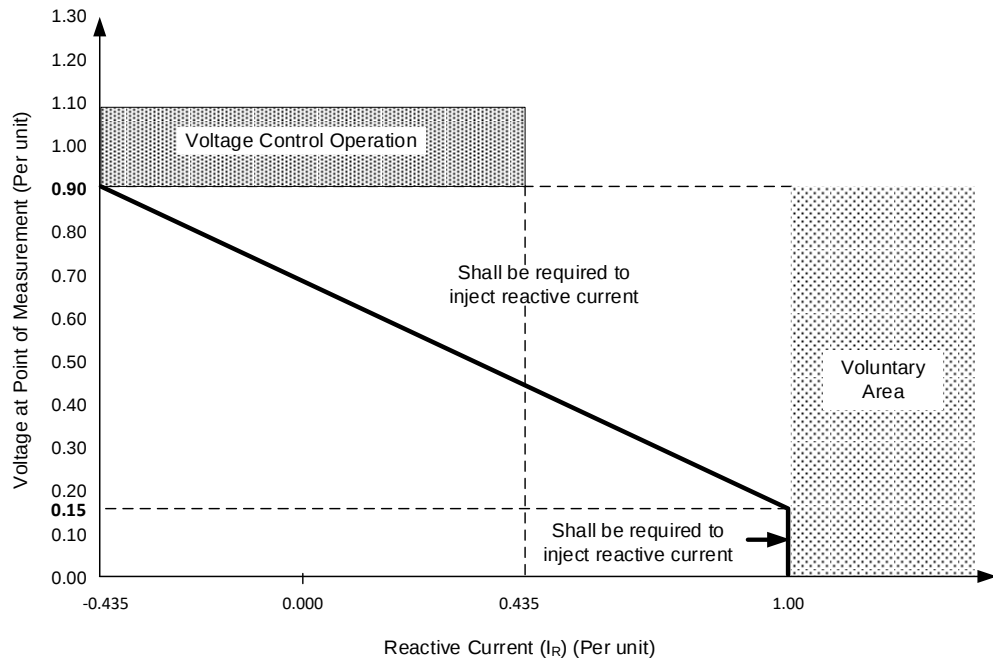
รูปที่ O-5 การควบคุมการจ่ายหรือรับ Reactive Current ของ โรงไฟฟ้าที่ใช้อุปกรณ์ Inverter
