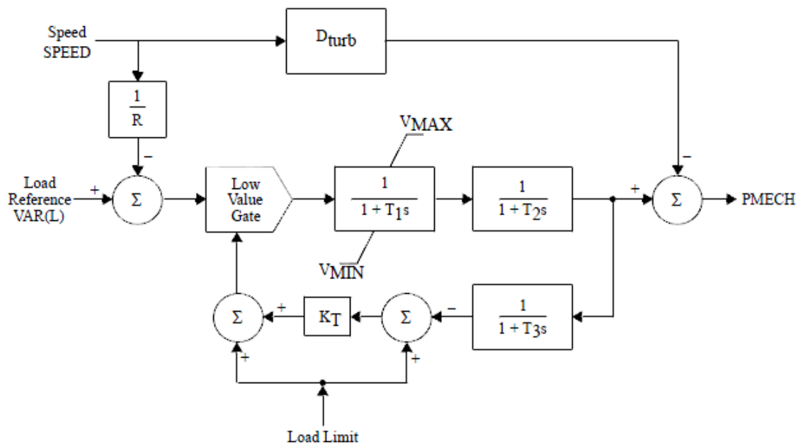
รูปที่ 1.1 ตัวอย่าง Block Diagram ของ GAST Model สำหรับ Gas Turbine-Governor
