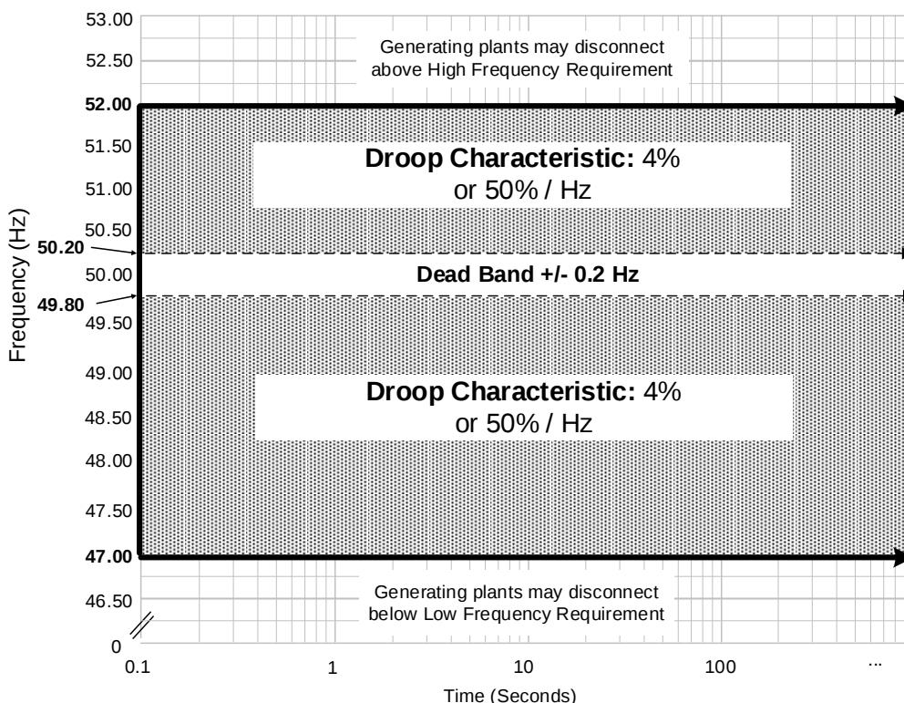
รูปที่ O-11 เกณฑ์ Frequency Ride Through ของ BESS
