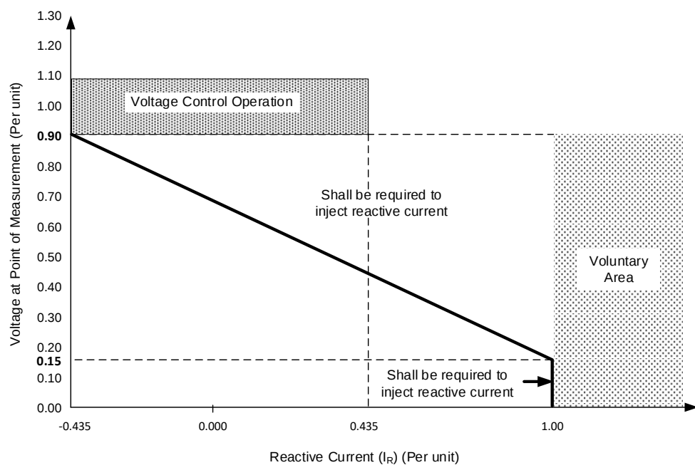
รูปที่ P-5 การควบคุมการจ่ายหรือรับ Reactive Current ของโรงไฟฟ้าที่ใช้อุปกรณ์ Inverter
