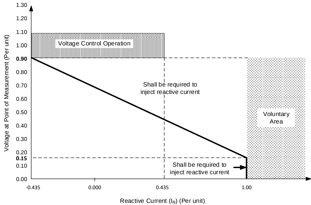
รูปที่ O-18 การควบคุมการจ่ายหรือรับ Reactive Current ของ โรงไฟฟ้าที่ใช้อุปกรณ์ Inverter
