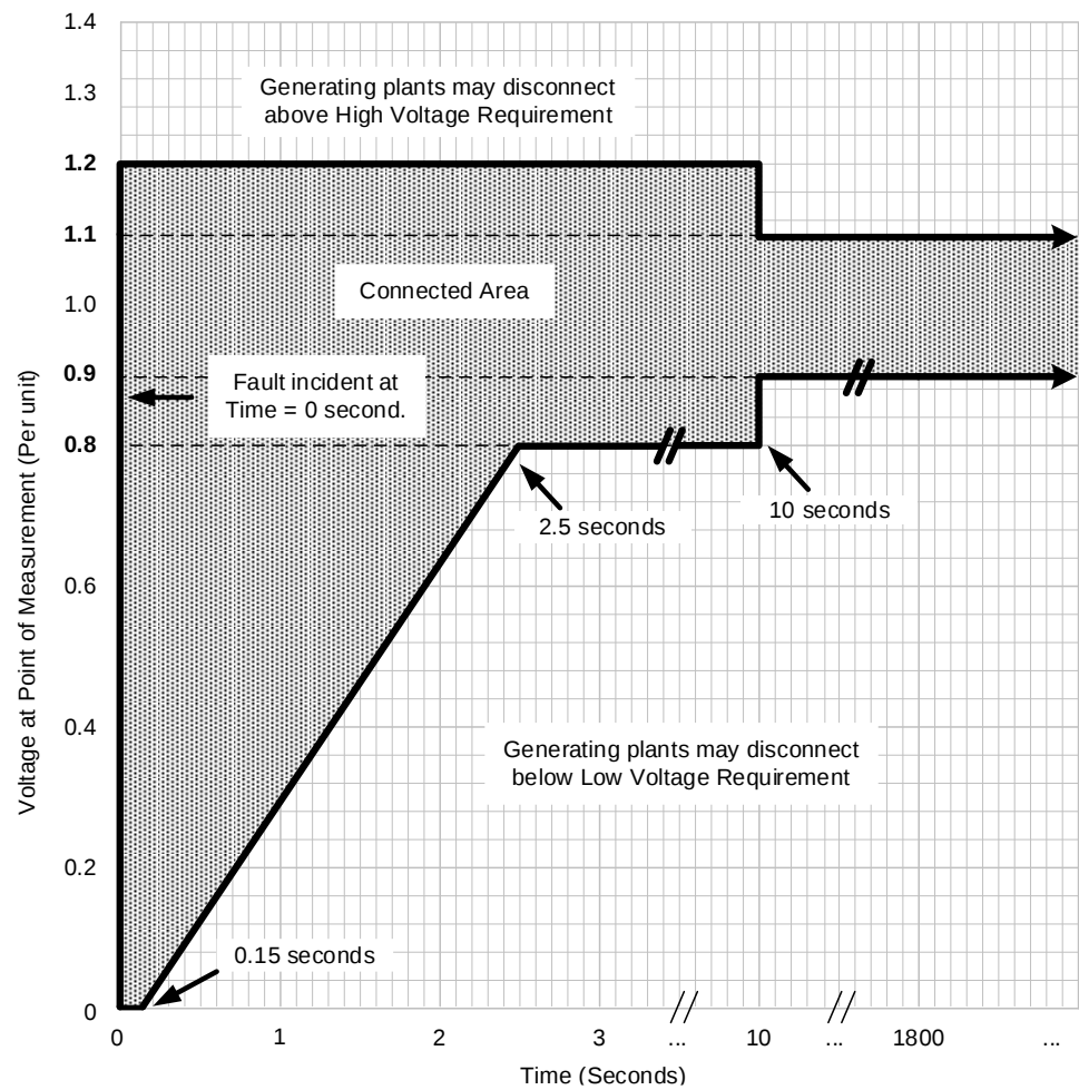
รูปที่ P-4 เกณฑ์ Voltage Ride Through ของโรงไฟฟ้าที่ใช้อุปกรณ์ Inverter
