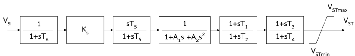
รูปที่ 1.3 ตัวอย่าง Block Diagram ของ PSS1A Model สำหรับ IEEE Stabilizing Model
