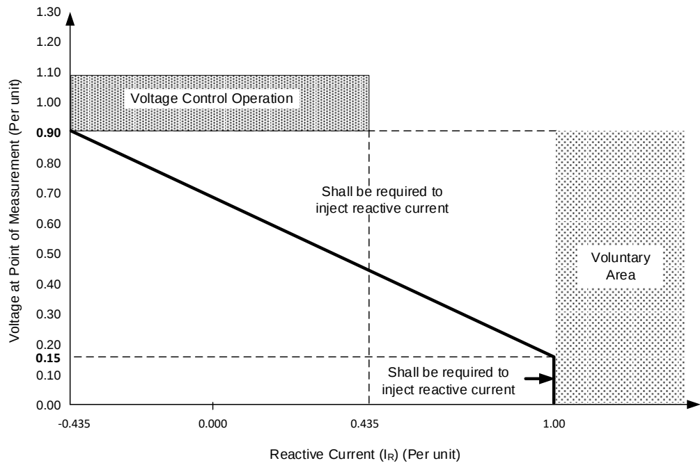
รูปที่ O-10 การควบคุมการจ่ายหรือรับ Reactive Current ของ โรงไฟฟ้าที่ใช้อุปกรณ์ Inverter
