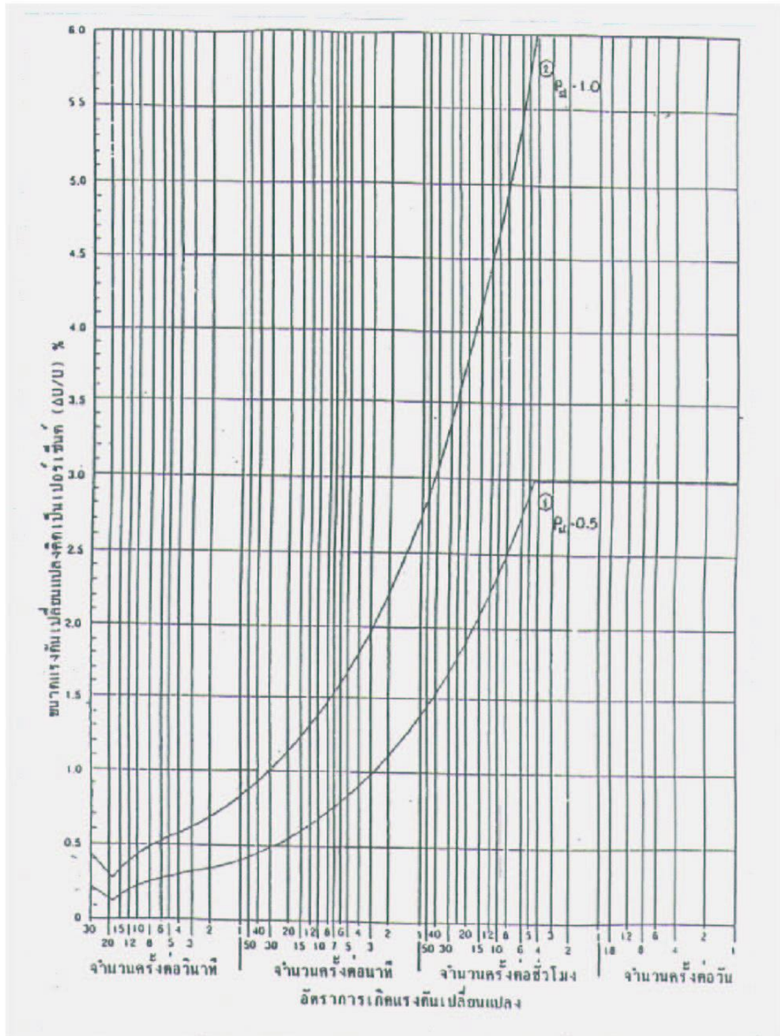
รูปที่ 5-1 รูปกราฟขีดจำกัดขนาดและอัตราการเกิดแรงดันผันแปลง
